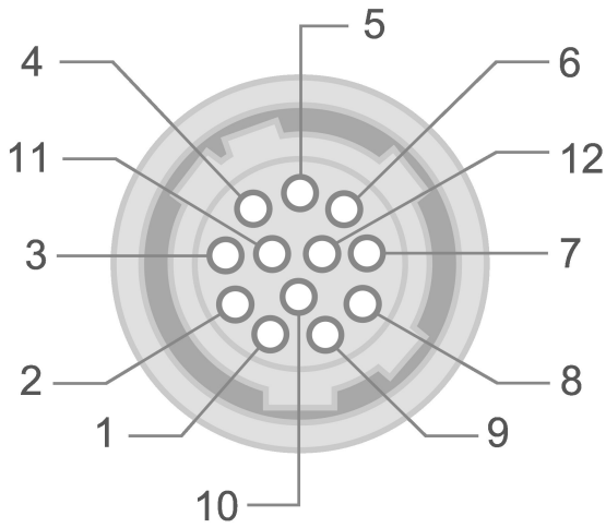
Cable side
